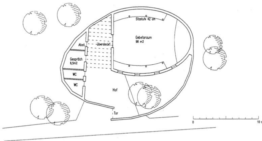
Gebetshaus Grundriss und Ansicht
